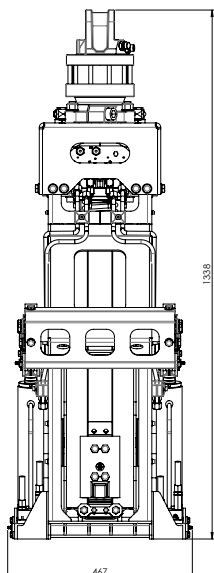
Speed-Gripper con adattatore a gancio, tipo VPV 020
