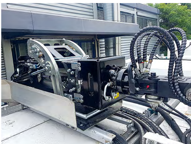
Il dispositivo di registrazione è in posizione di riposo
