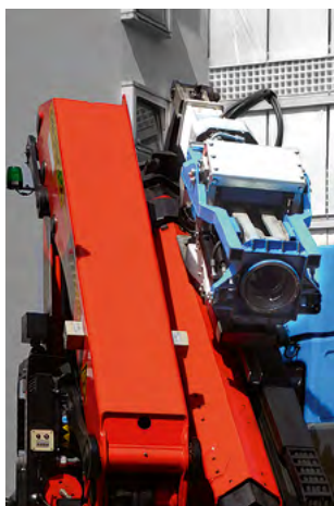
Dispositivo di sollevamento comprensivo di freno a pendolo e bilancia radio per gru
