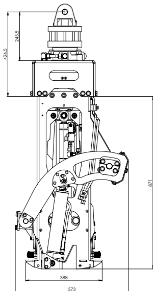
Speed-Gripper con adattatore a gancio, tipo VPV 020
