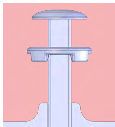
Rondella a fungo fissa con nervature di bloccaggio, 32 mm
